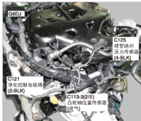
228. 发动机后部
