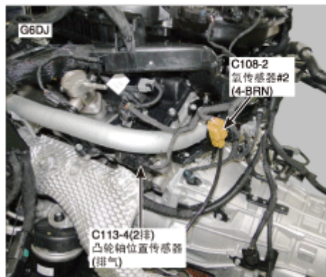
223. 发动机后部
