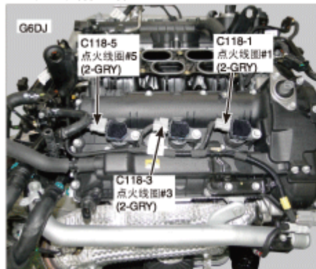
226. 发动机右侧上部
