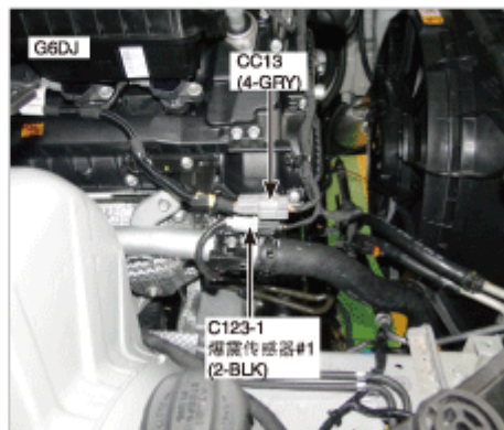
225. 发动机右侧上部
