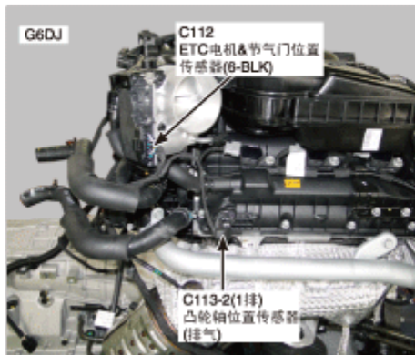
227. 发动机右侧上部
